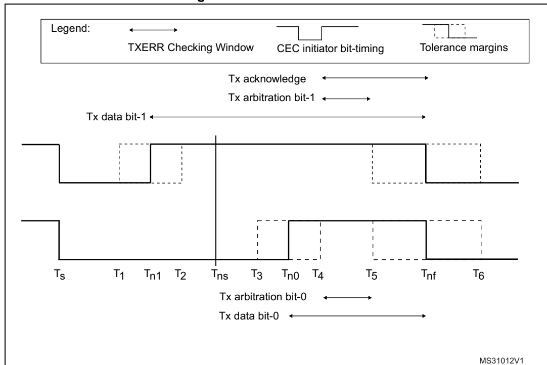
Figure 338. TXERR detection
